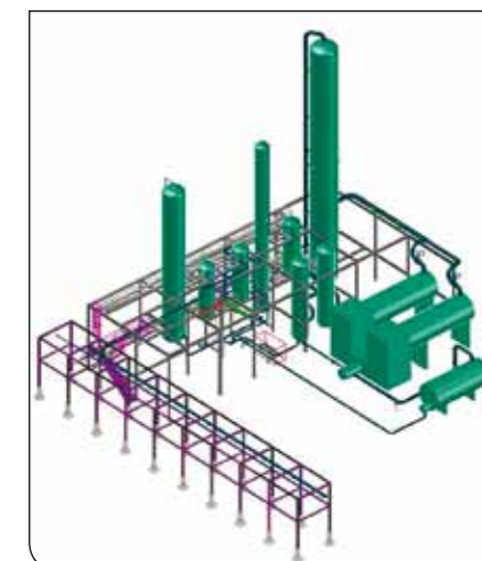
Portion d'une usine chimique modélisée dans CADWorx Plant Professional.
